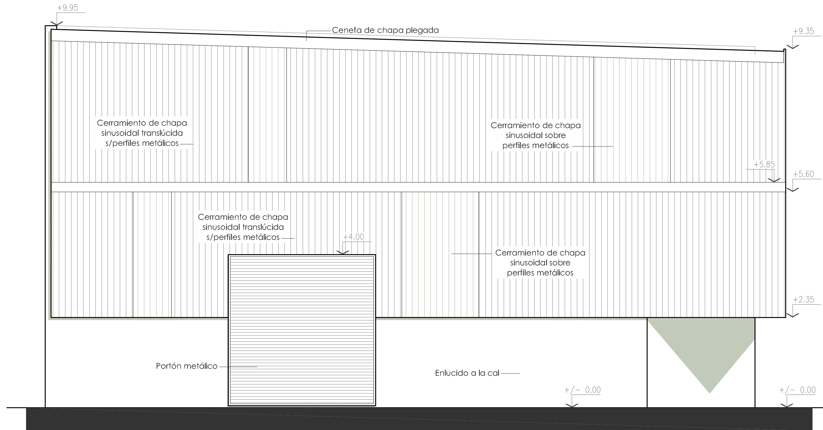
FACHADA ESTE esc 1 100
