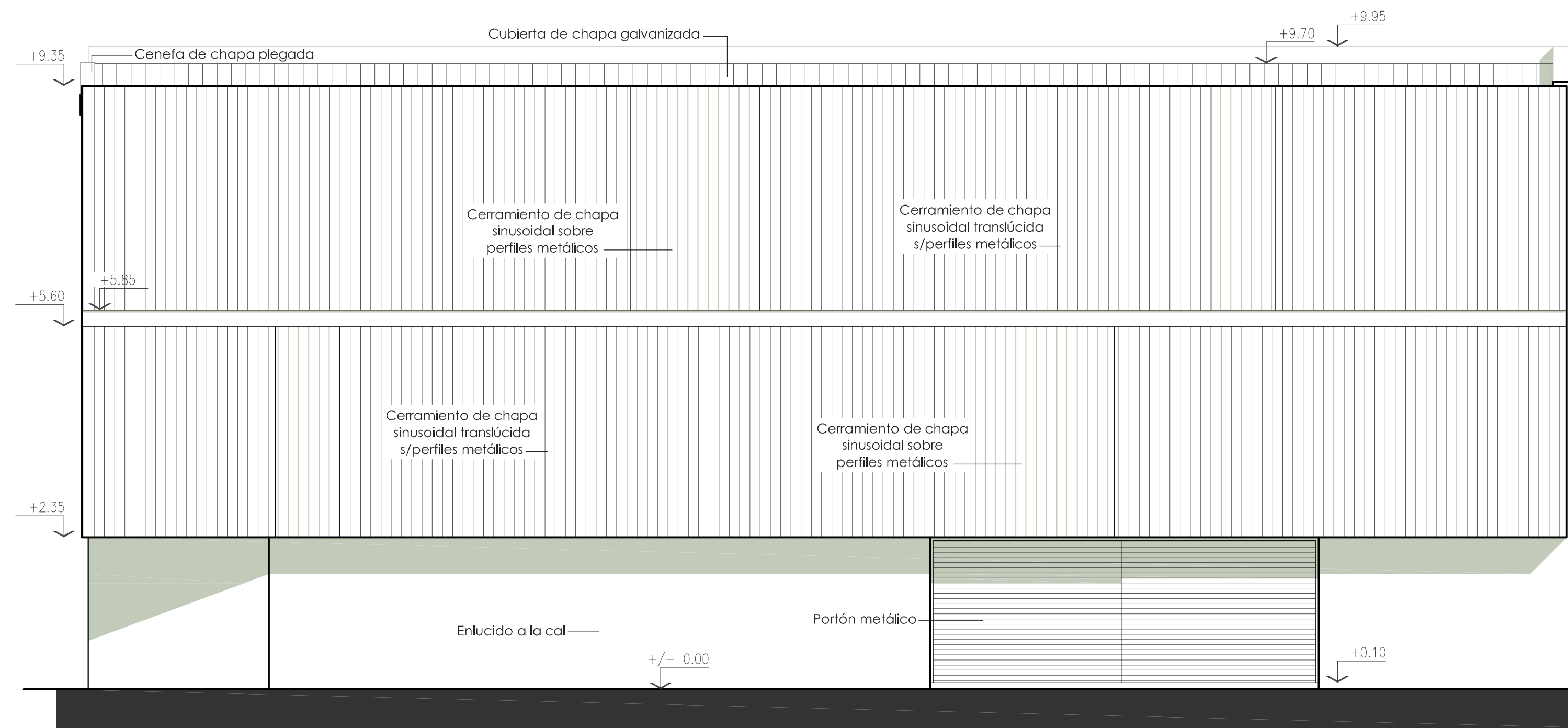
FACHADA NORTE esc 1.100
